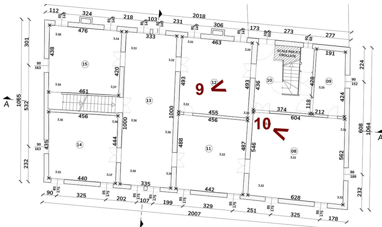
Piano primo
